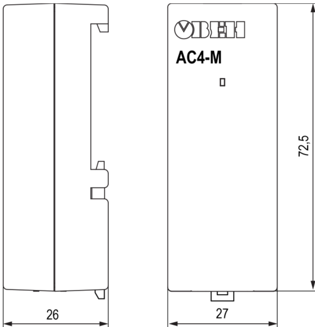
Рисунок 1 - Габаритные размеры
