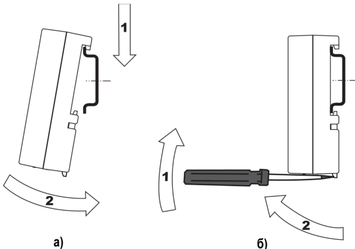
Рисунок 2 – Монтаж и демонтаж
