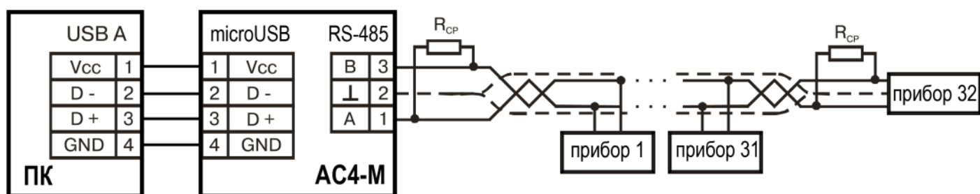
Рисунок 3 - Схема подключения прибора
